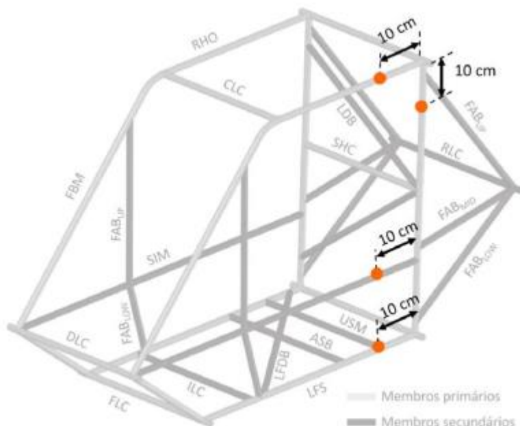
Figura 1: Posições onde deve ser realizada a furação
