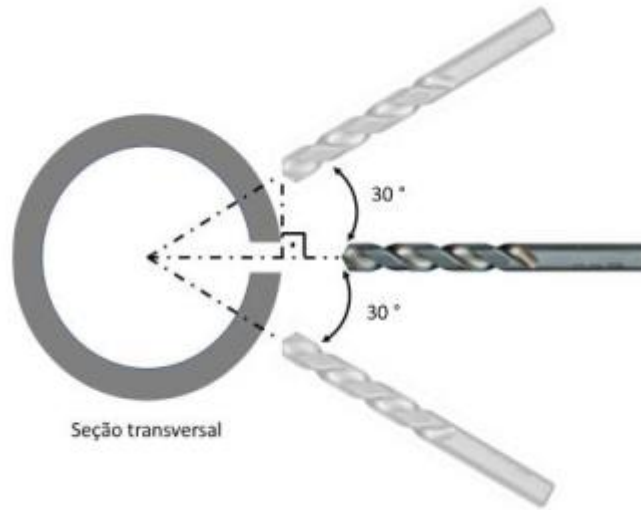
Figura 2: Diagrama demonstrando como o furo deve ser executado
